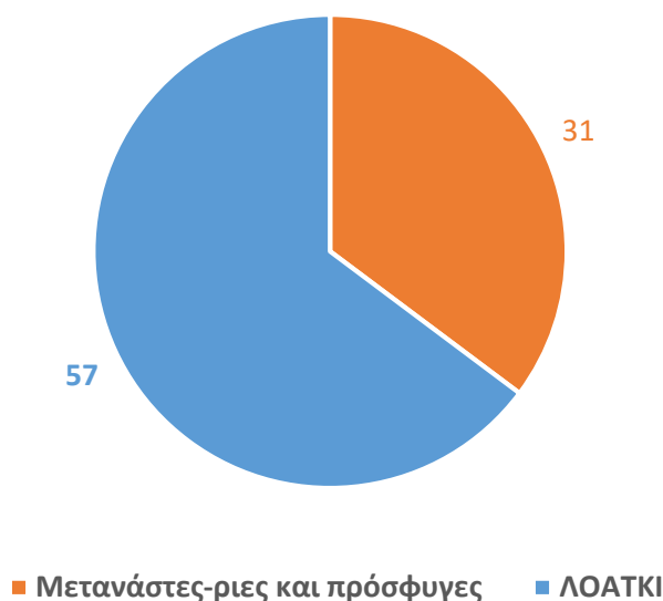
Λόγος στοχοποίησης
